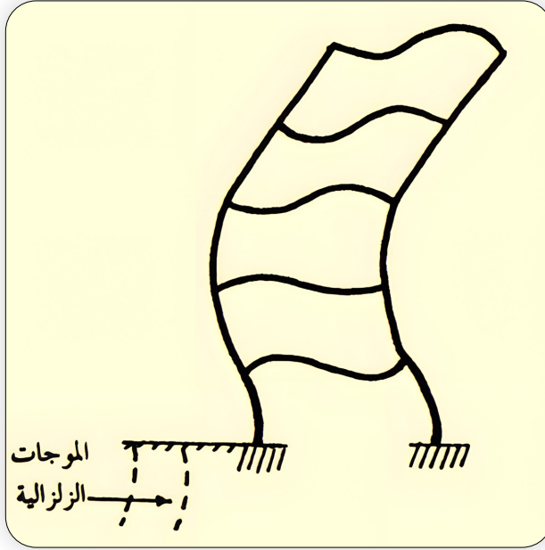
شكل (١٦): تأثير الموجات الزلزالية على المبنى ككل.
