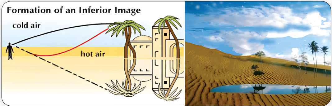
شكل (٢١): التفسير العلمي للسراب كظاهرة موجودة في الطبيعة.
