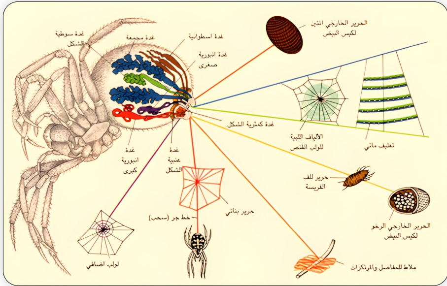
شكل (١٢): سبع غدد مختلفة في رأس أنثى العنكبوت لإنتاج سبعة أنواع مختلفة من الخيوط الحريرية.
